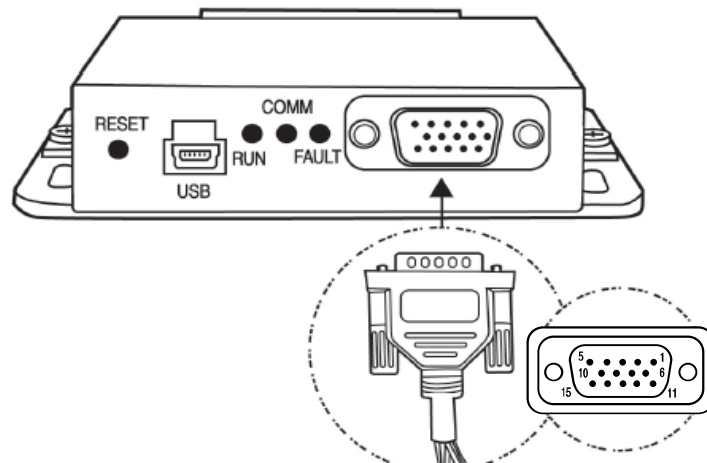
그림 4 D-Sub Female 커넥터 연결
