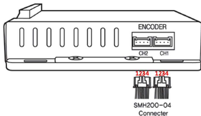
그림 3 엔코더 커넥터 연결
