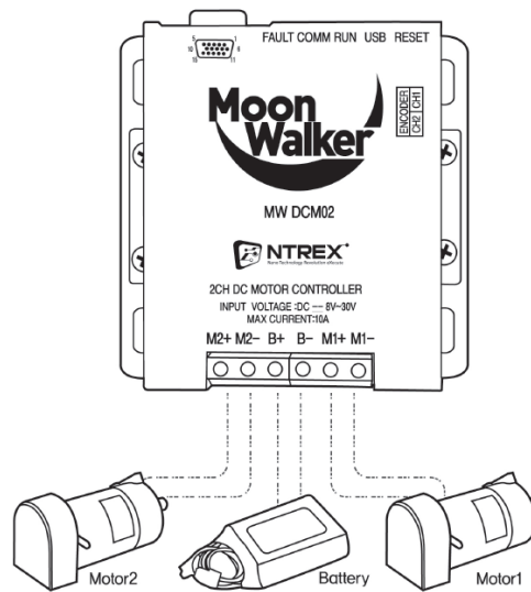
그림 1 전원 및 모터 연결
